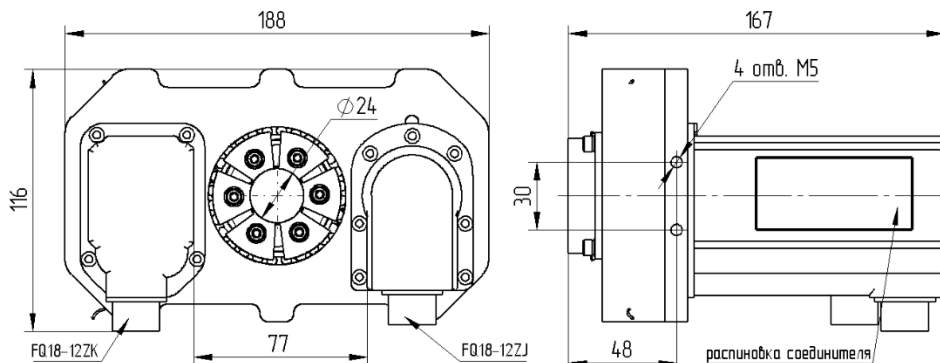
Рисунок 1 – Общий вид и габариты изделия.
